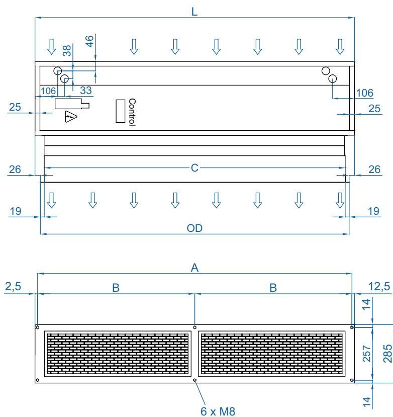
Instal·lació horitzontal
